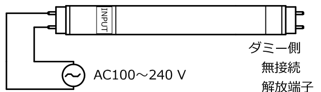
配線図 AC電源接続側 INPUT 表示シール有り 片側給電
