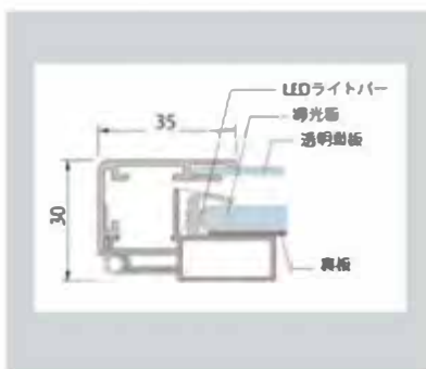
アルミフレーム断面略図
