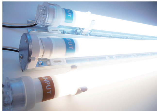
AC100 ~ 240V、20・30・32・40 w型 (昼光色、電球色)。照度 2300 lm以上 (40 w型)、飛散防止フィルム加工。推奨看板厚は 150 mm以上。
