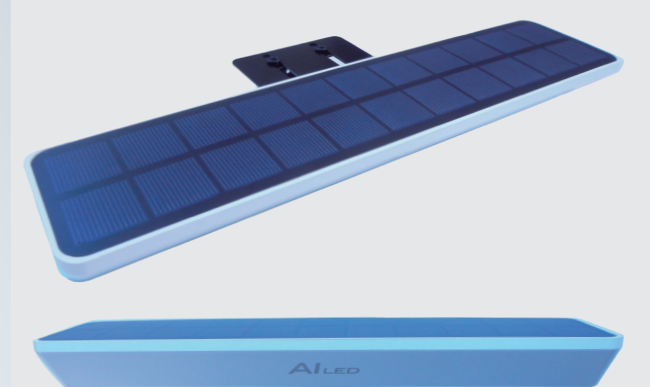
W285 x H70 x D30 mm、昼光色 6000k / 電球色 3000k、IP65 (防水)。推奨：A型看板用や住宅用表札・ポストなど。
